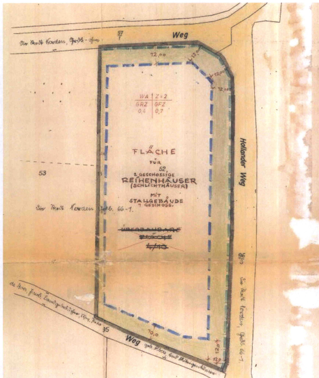
Bebauungsplan Nr. 3 (Auszug), unmaßstäblich
